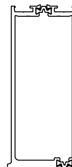
TB D23 BEVEL STILE CONTINUOUS HINGE
