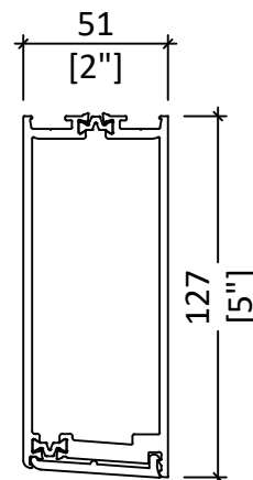
TB D22 BEVEL STILE BUTT HINGE AND LOCK SIDE
